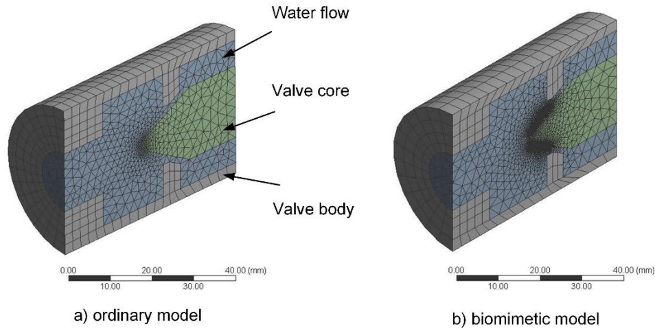
Fig. 5. Meshing
